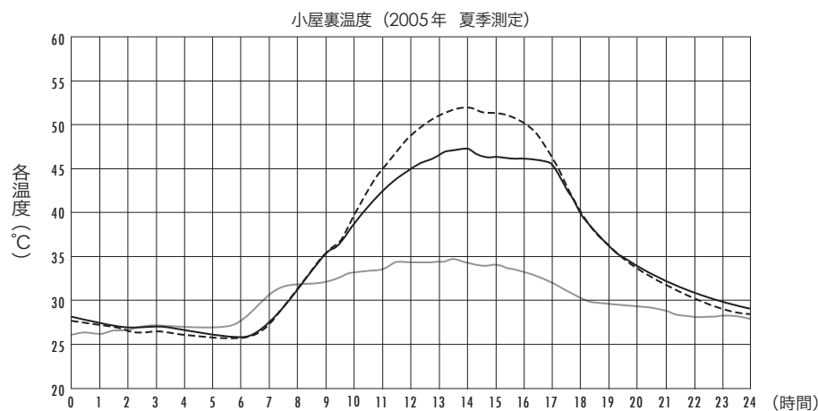
●小屋裏温度 (夏季晴天日での温度変化)
